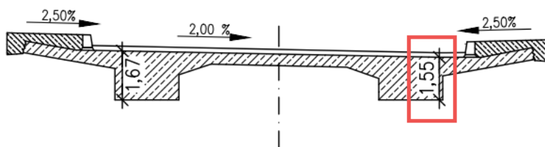
Schnitt B-B
