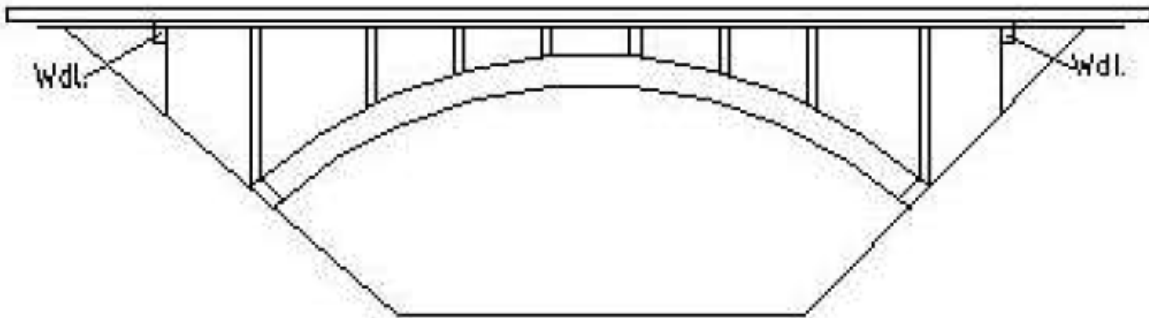
Abbildung 1: Struktur eines Bogens mit aufgeständerter Fahrbahn gem. Anhang D7 der ASB-ING
